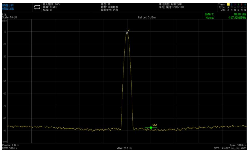
图 3-20: 相位噪声
