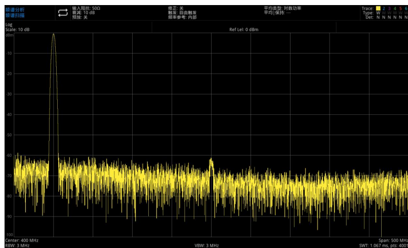
图 3-16 谐波失真
