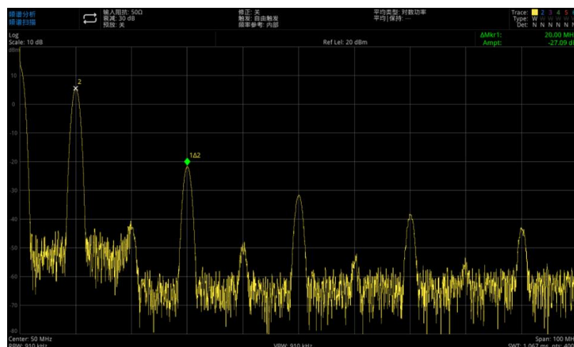
图 3-2：标记模式差值 \Delta 在同一屏幕信号比较
