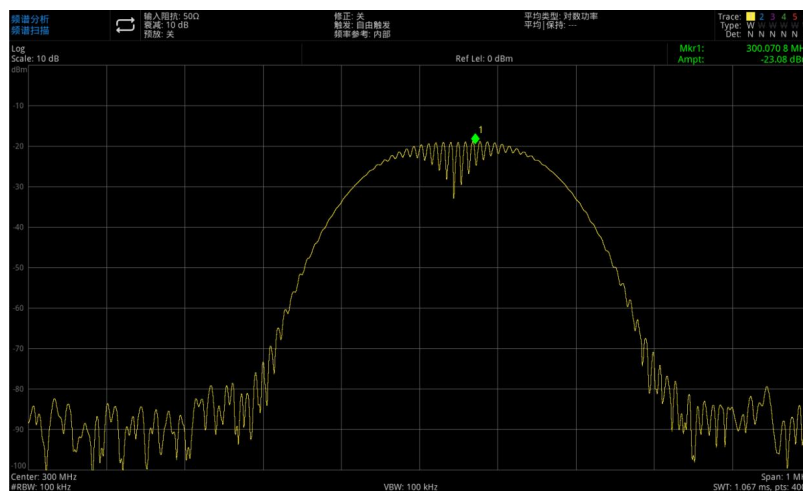
图 3-5：没有分辨出的两个等幅信号
