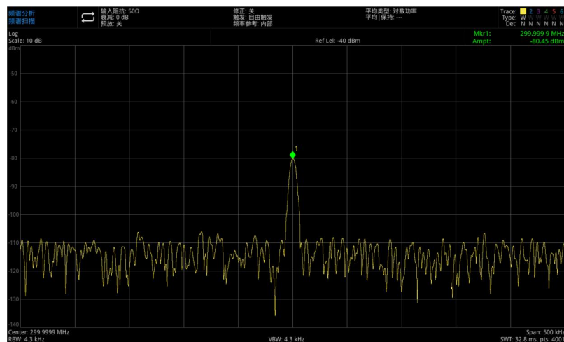
图:3-12: 在 0dB 衰减下测量小信号
