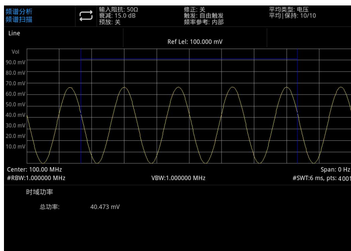
图 5-2：时域功率
