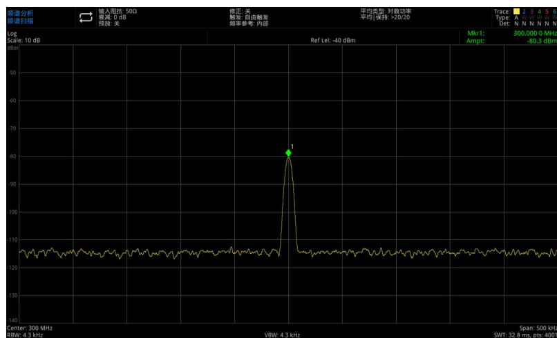
图 3-14：迹线平均
