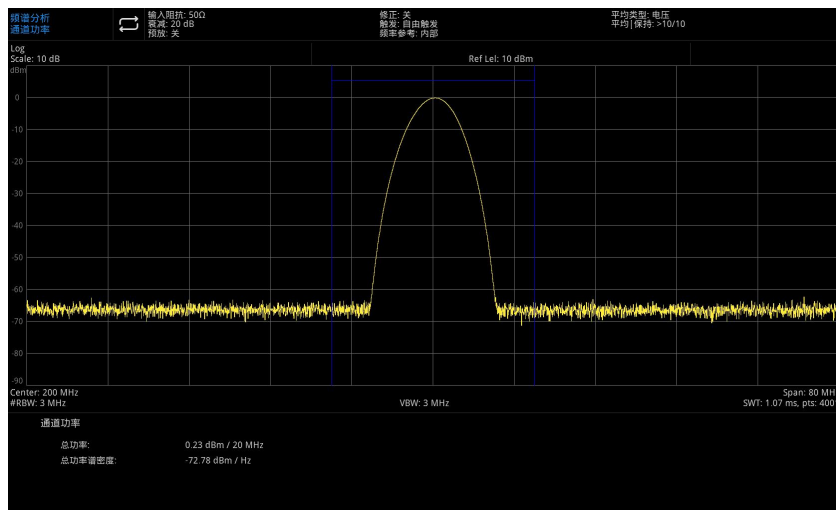
图 5-1: 通道功率
