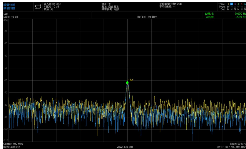
图 3-17 谐波失真分量
