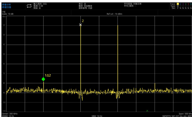
图 3-19: 测量失真产物
