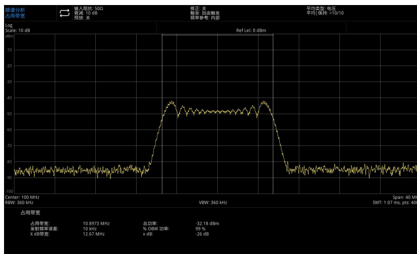
图 5-3:占用带宽
