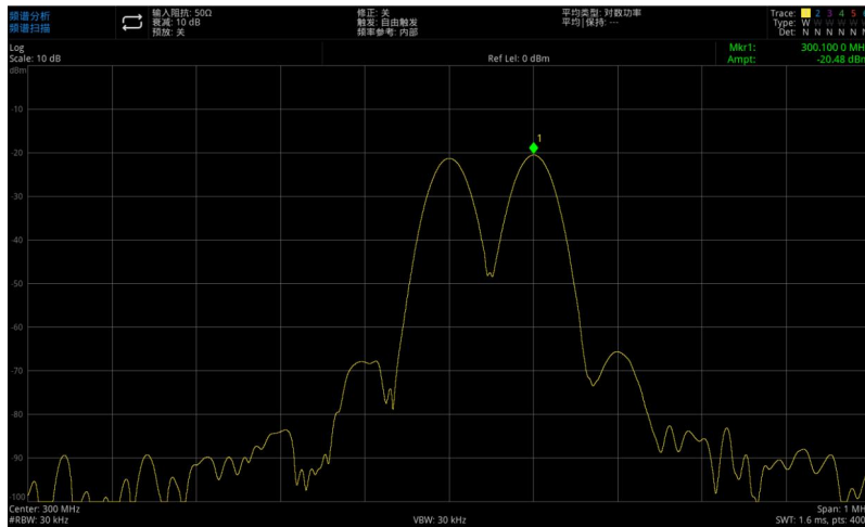
图 3-6: 分辨出的两个等幅信号 (1)
