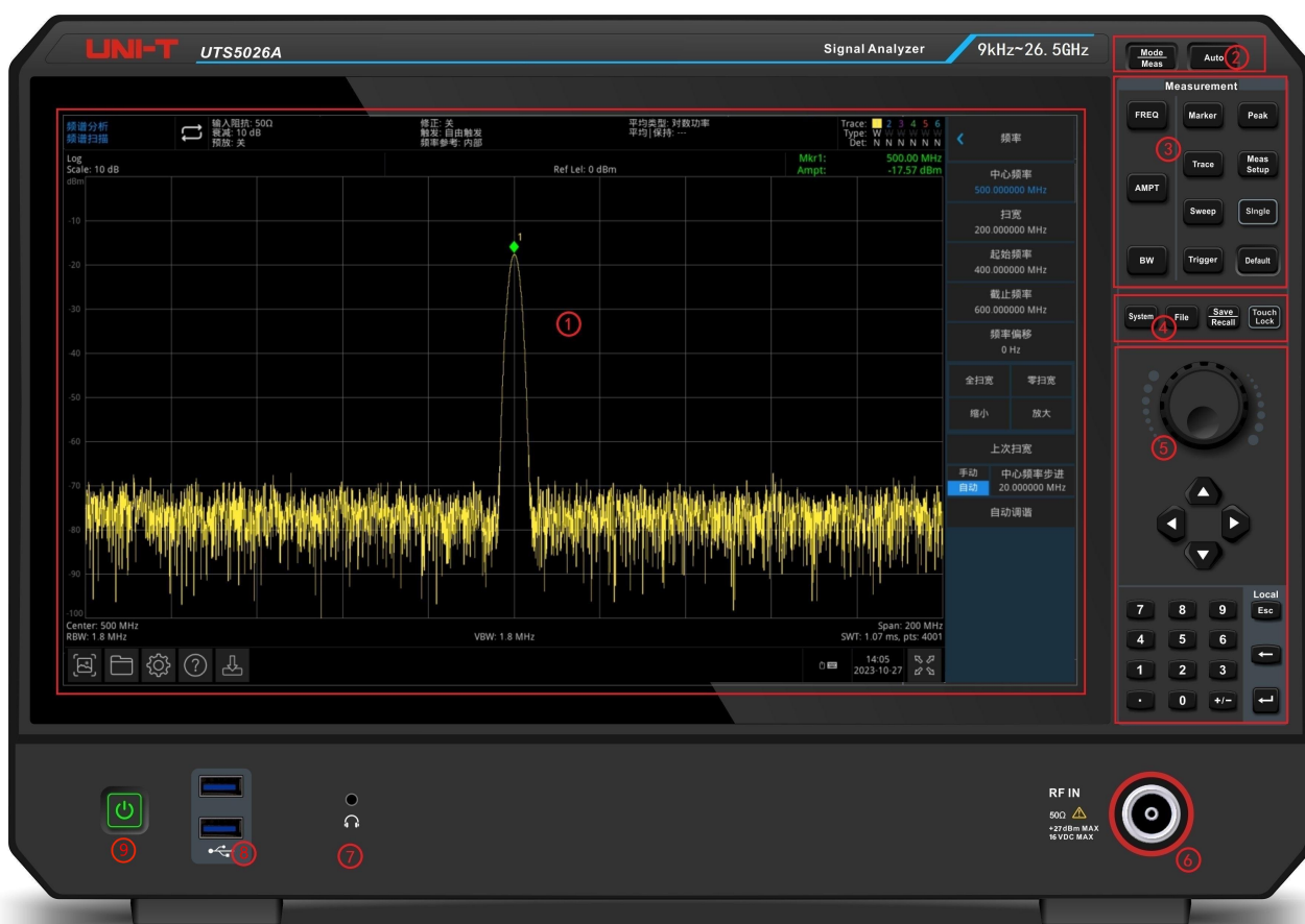
图 1-1: 前面板
