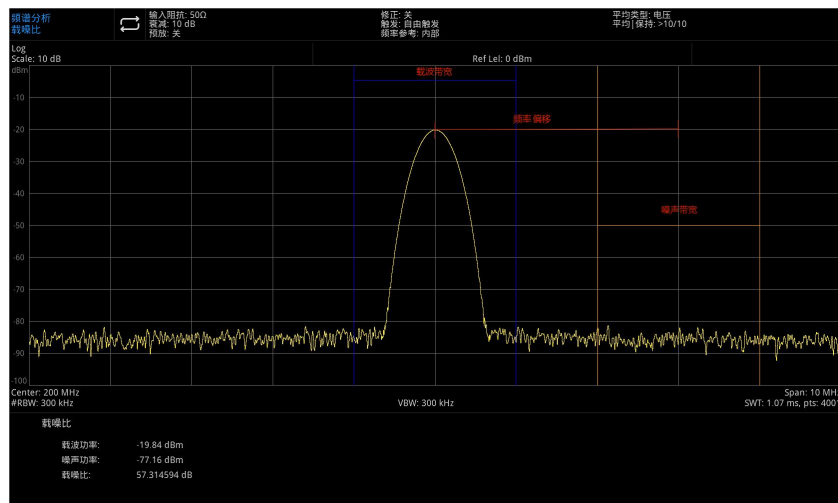
图 5-7：载噪比测量
