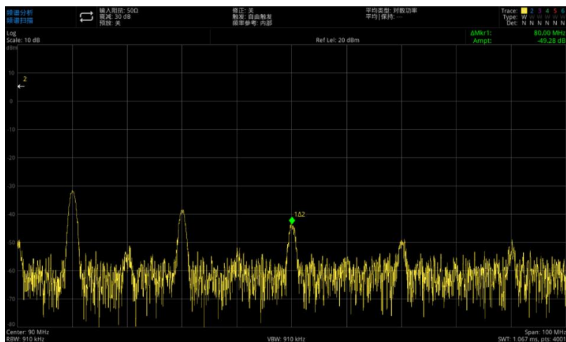
图 3-3：参考信号在屏幕外的 Delta 标记
