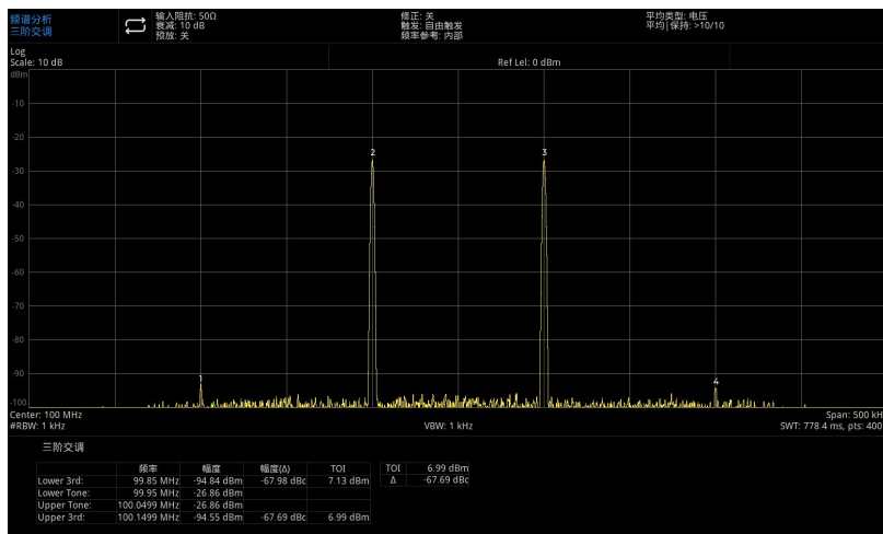
图 5-4: 三阶交调
