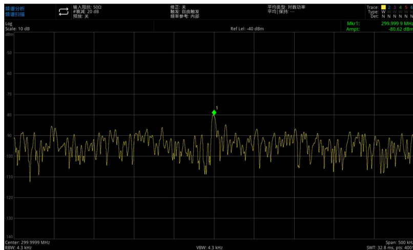
图 3-11: 接近底噪的信号
