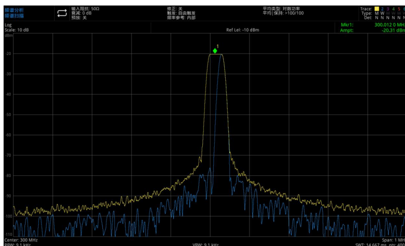
图 3-15: 用最大保持和刷新来观察信号漂移
