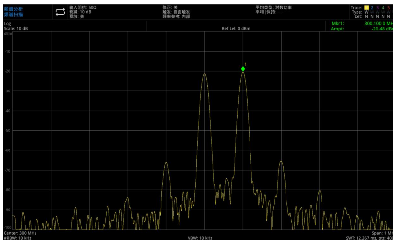
图 3-7: 分辨出的两个等幅信号 (2)
