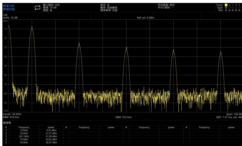
图 4-3：峰值表
