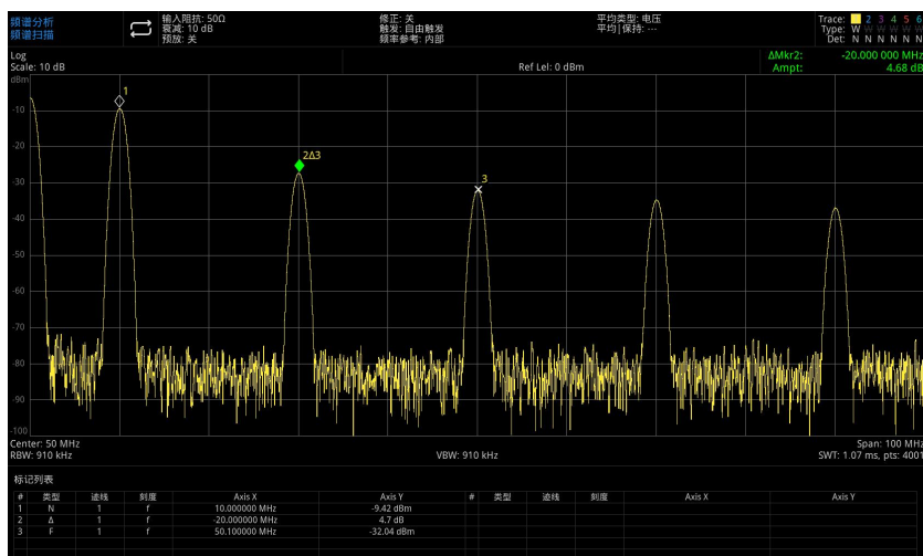
图 4-2: 标记列表
