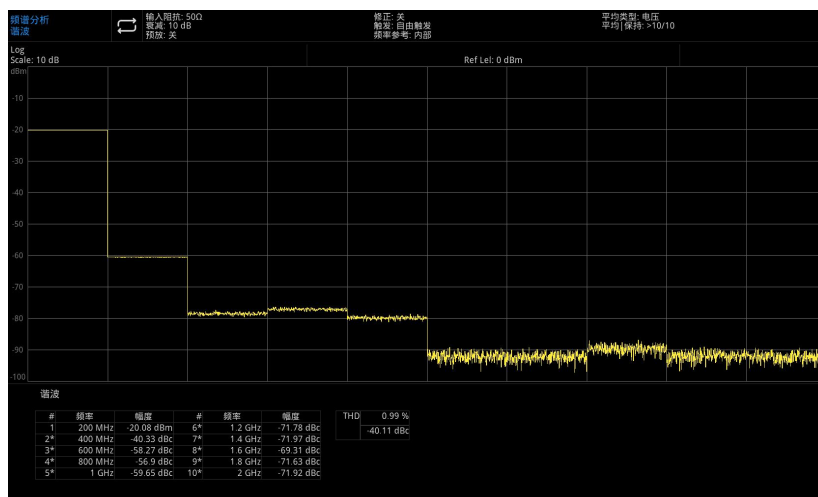
图 5-8: 谐波测量
